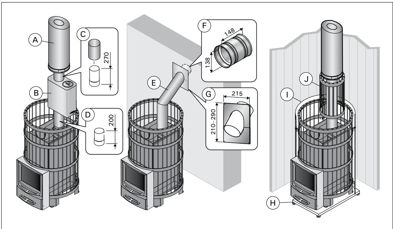
Kuva 15. Lisätarvikkeet (mitat millimetreinä) Bild 15. Tilläggsutrustning (mått i millimeter)
